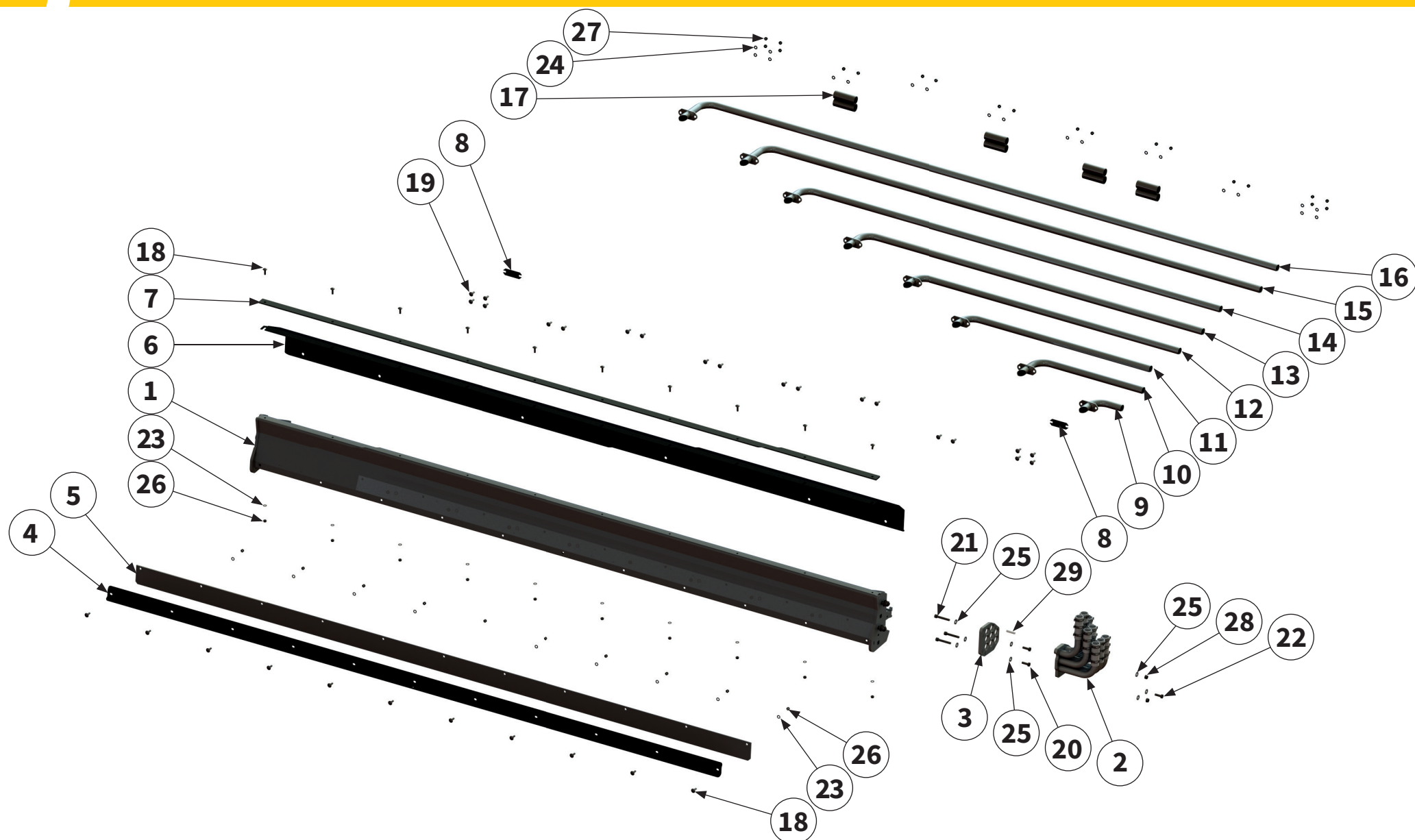
SAATZUFUHR GEHÄUSE LINKS | Left-hand seed feed housing | Alimentation en semences Carter gauche | Carcasa izquierda de alimentación de semillas
